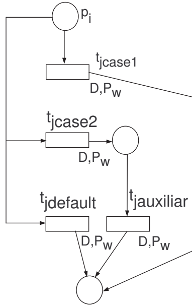
Figura 4.3 Exemplo da Rede de Petri do Switch
