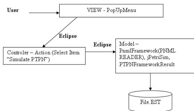
Figura 5.3 Simulador da Power Petri Net Estocástica - Plugin Schema
