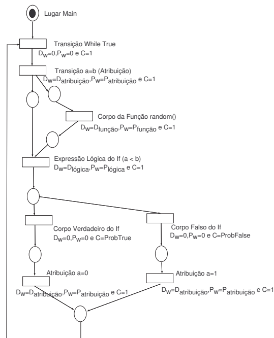
Figura 4.9 Exemplo da Composição das Estruturas Básicas
