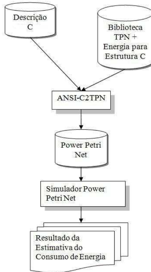
Figura 3.1 Visão Geral da Arquitetura da Power Petri Net
