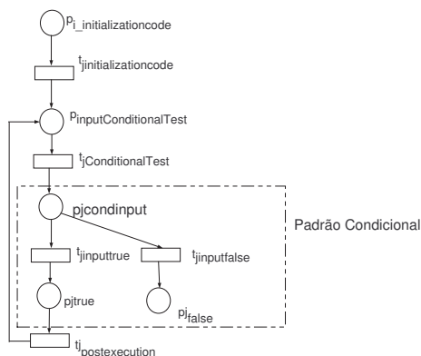
Figura 4.4 Exemplo da estrutura de Iteração FOR, composta pelos padrões Seqüencial e Condicional
