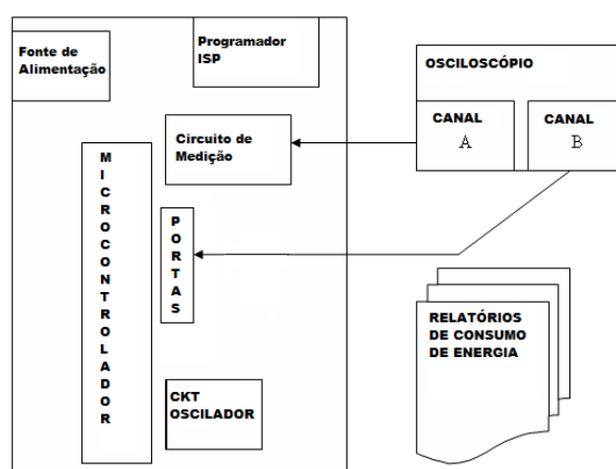
Figura A.2 Hardware usado para Caracterização do Processador - Medição Tempo e Potência(Energia)
