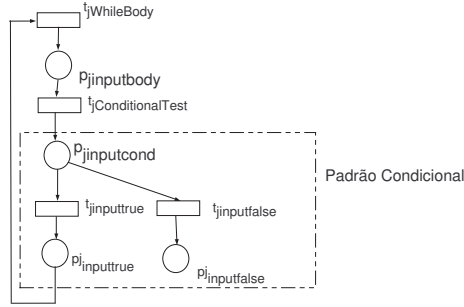
Figura 4.5 Rede de Petri da Iteração Do-While
