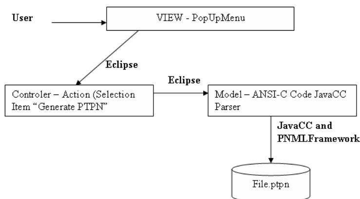
Figura 5.1 Arquitetura do Parser de ANSI-C para PTPN
