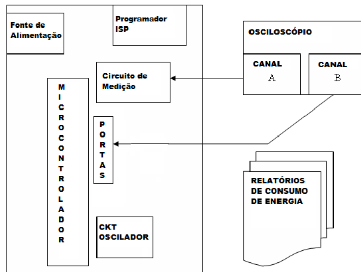
Figura 3.2 Hardware usado na Caracterização do Processador
