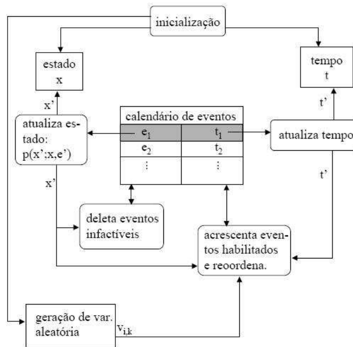
Figura 2.8 Exemplo de um Sistema de Escalonamento de Eventos
