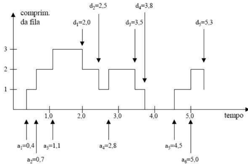
Figura 2.12 Diagrama dos eventos chegarão e partirão da fila como dados de entrada da simulação
