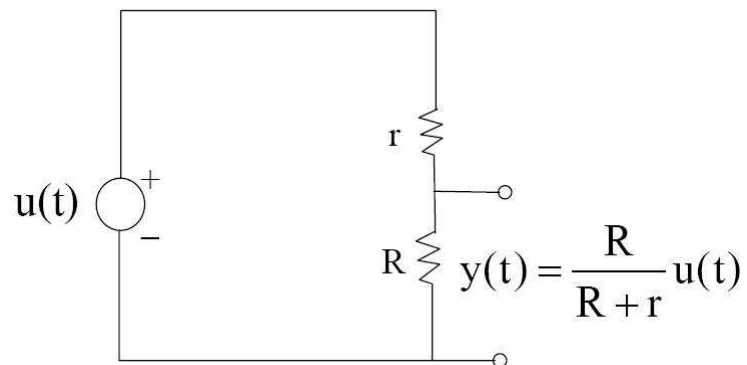
Figura 2.2 Modelo de um Circuito Elétrico
