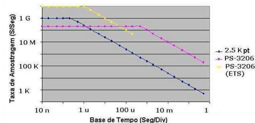
Figura A.3 Efeito da limitação de memória na redução da taxa de amostragem.
