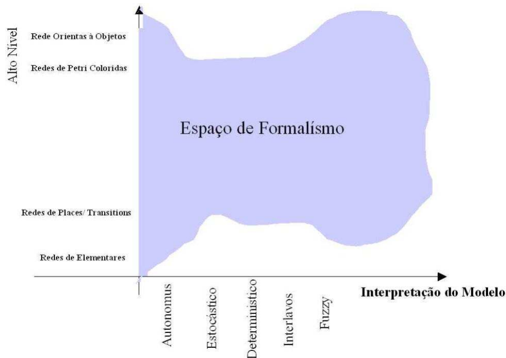
Figura 2.7 Abstração X Interpretação.
