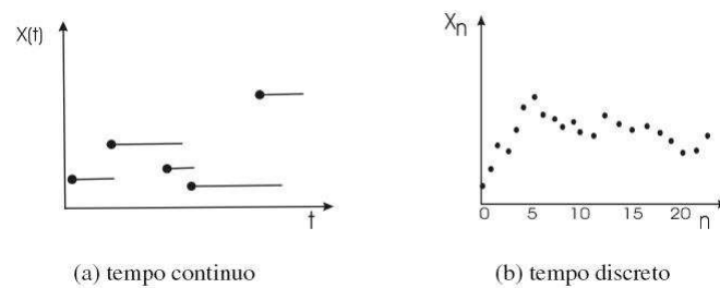
Figura 2.4 Amostras de Processos Estocásticos
