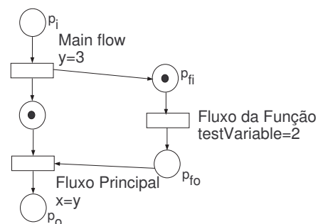
Figura 4.7 Rede de Petri para uma chamada de função
