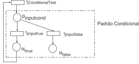
Figura 4.6 Rede de Petri da Iteração While
