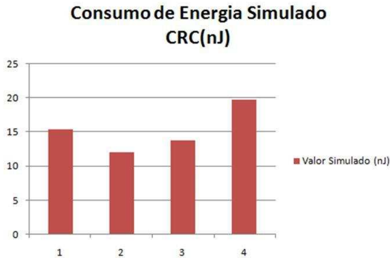
Figura 6.3 Gráfico da Estimativa de Consumo de Energia do CRC
