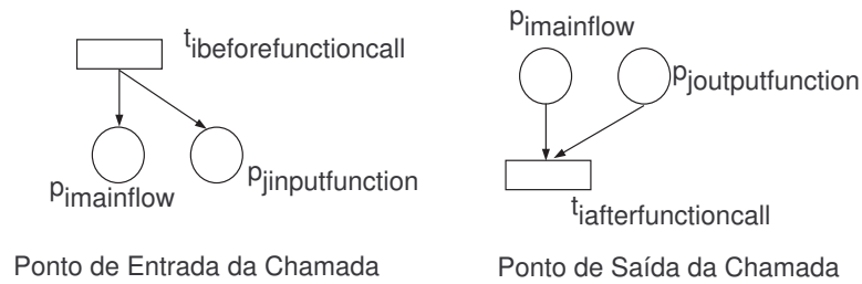
Figura 4.8 Rede de Petri com o Padrão de Chamada de Função
