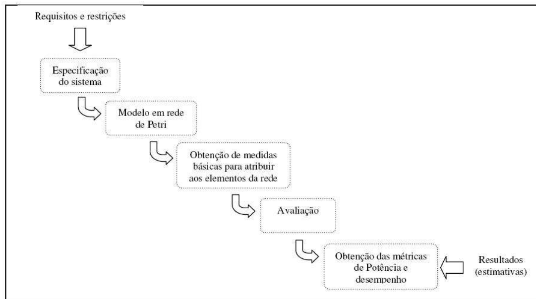
Figura 1.3 Atividades que compõem a metodologia proposta por [8]
