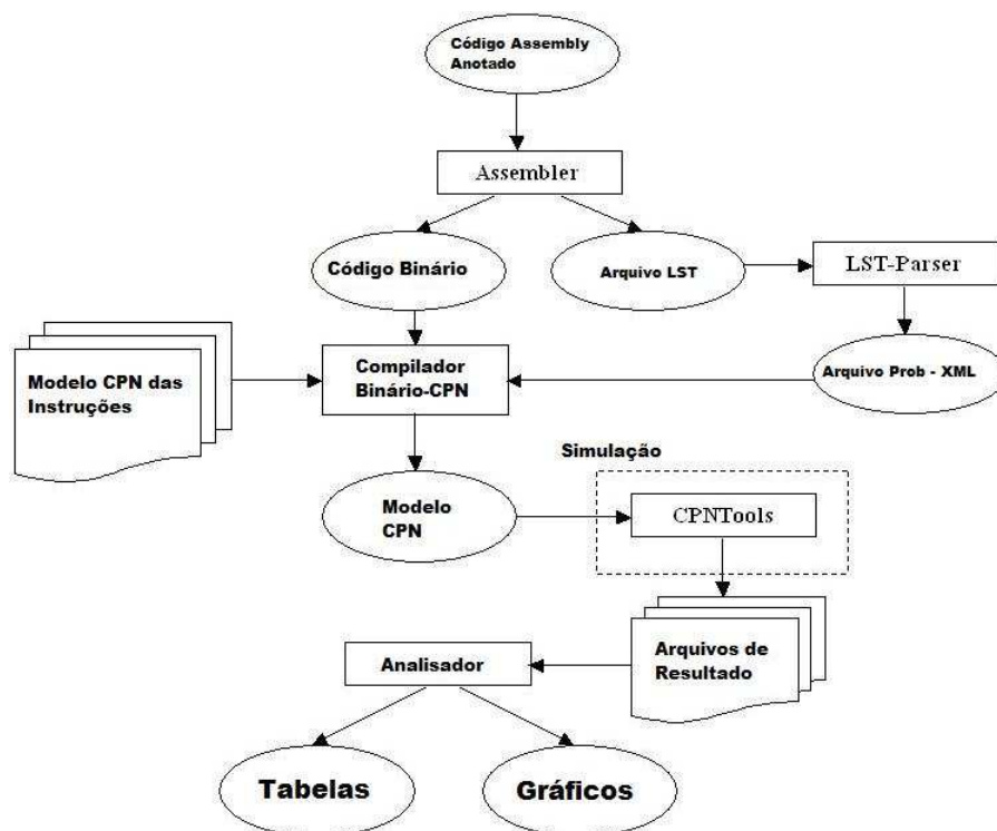
Figura 1.1 Framework Proposto pelo trabalho [7]
